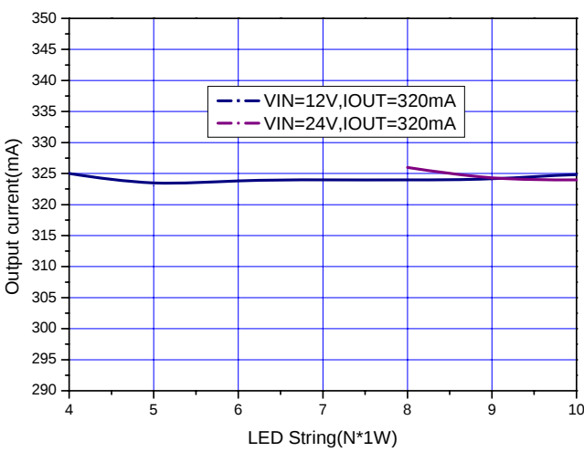
线性与负载调整率：
