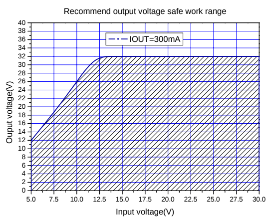
Figure7.Max output voltage(IOUT=300mA)
