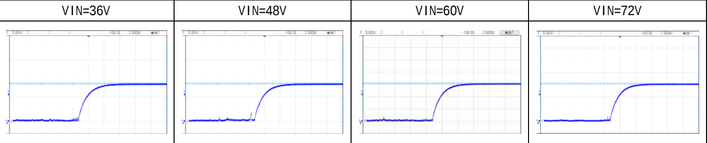
蓝色通道：输出电压波形，5V/格；秒格：2mS/格。
