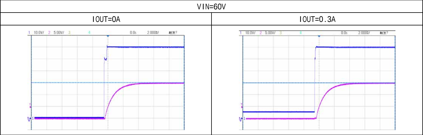
蓝色通道：输入电压波形，10V/格；紫色通道：输出电压波形，5V/格；秒格：2mS/格。
