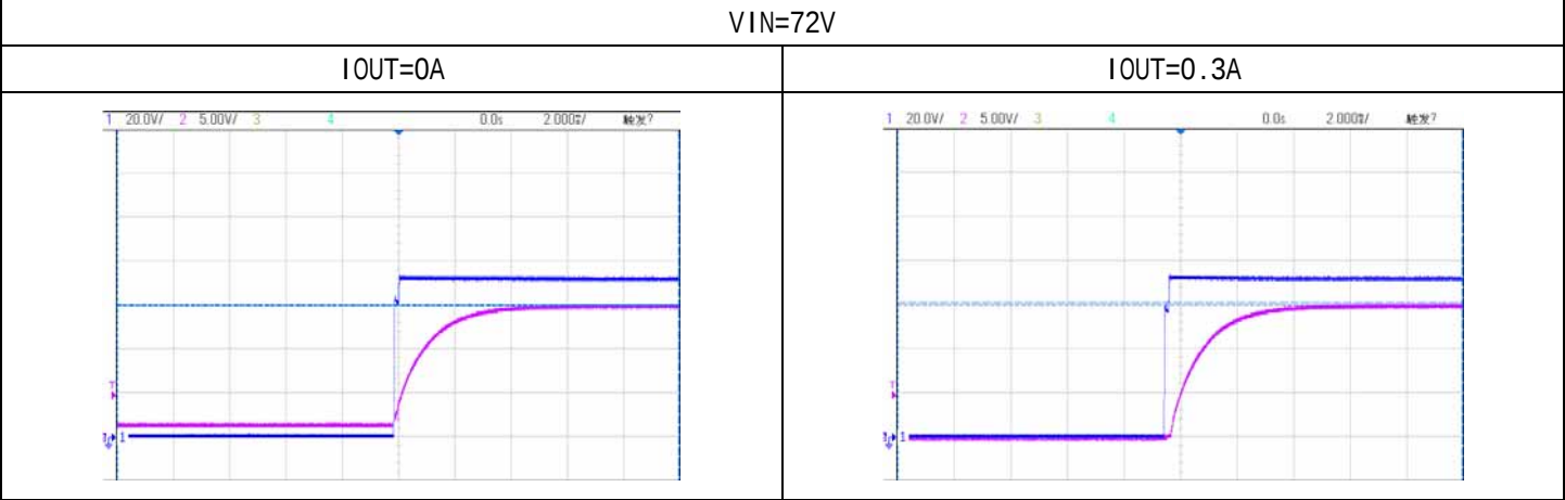
蓝色通道：输入电压波形，20V/格；紫色通道：输出电压波形，5V/格；秒格：2mS/格。
