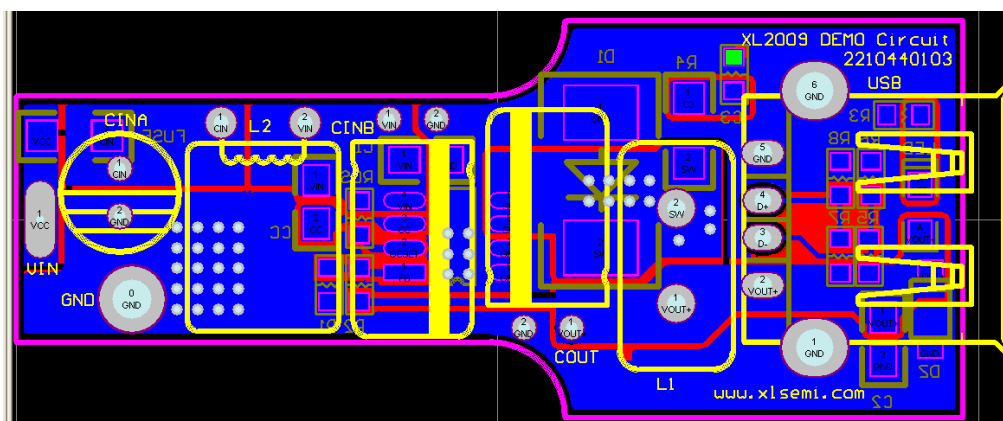
底层
